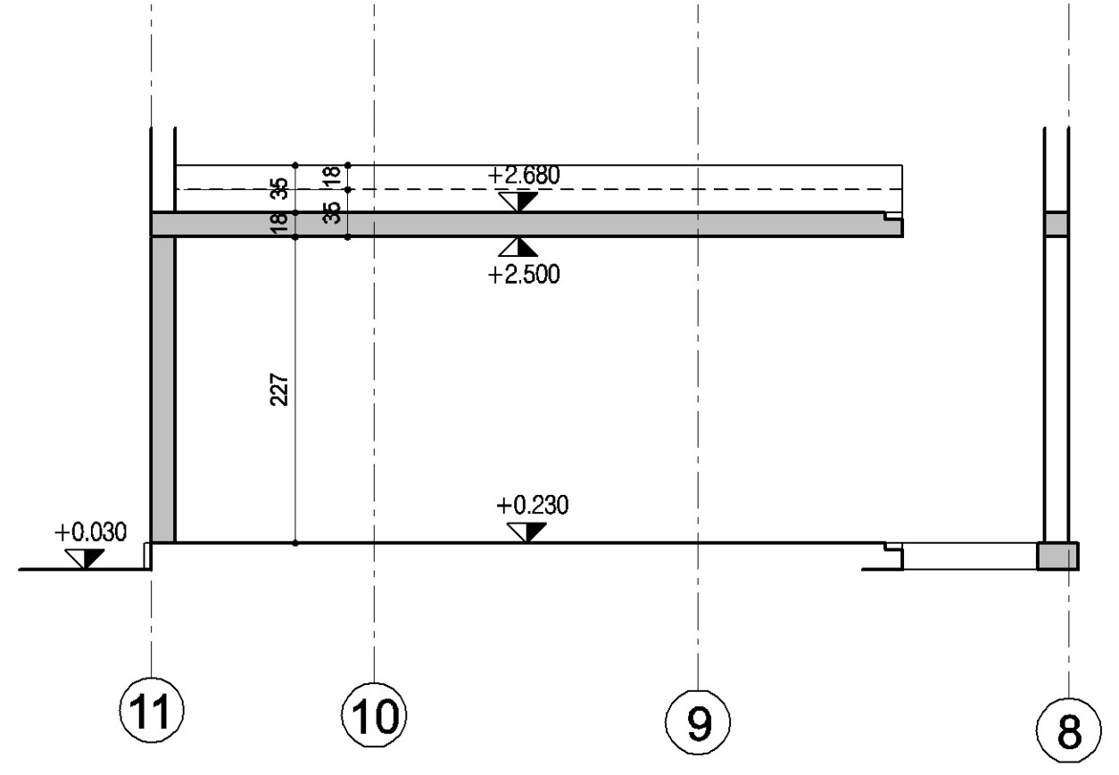
SCHNITT 4-4
