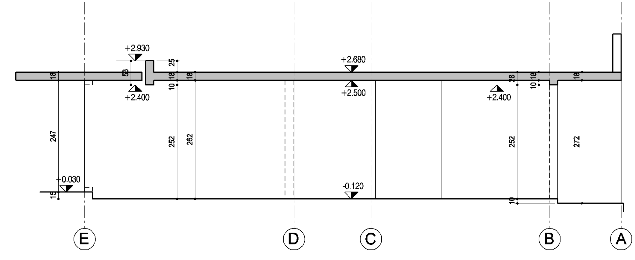
SCHNITT 8-8
