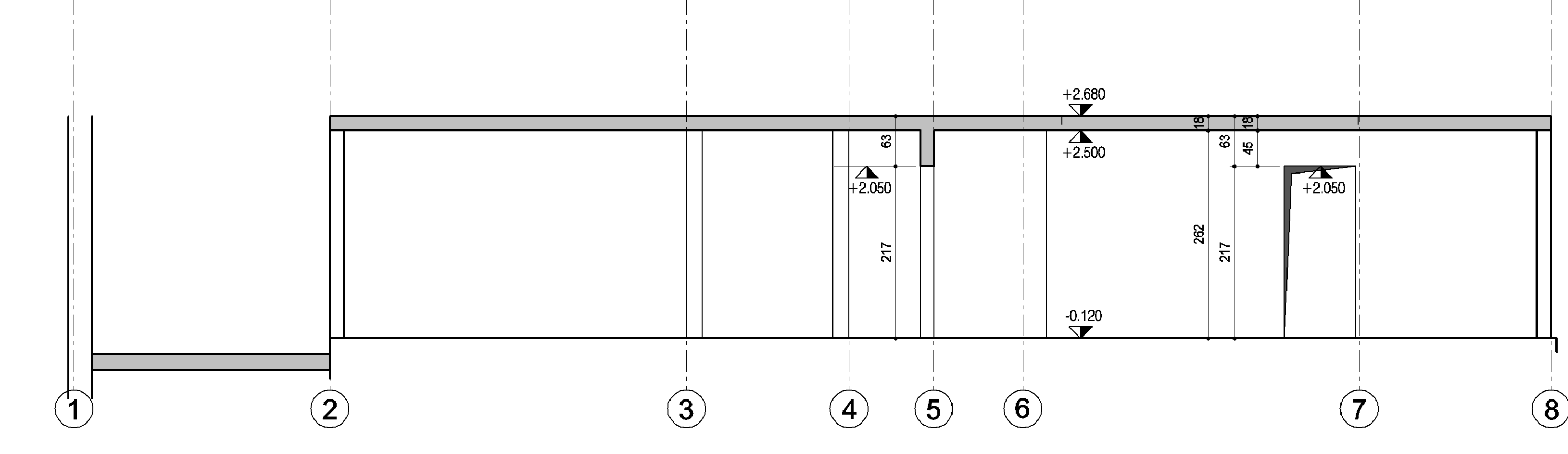
SCHNITT 3-3
