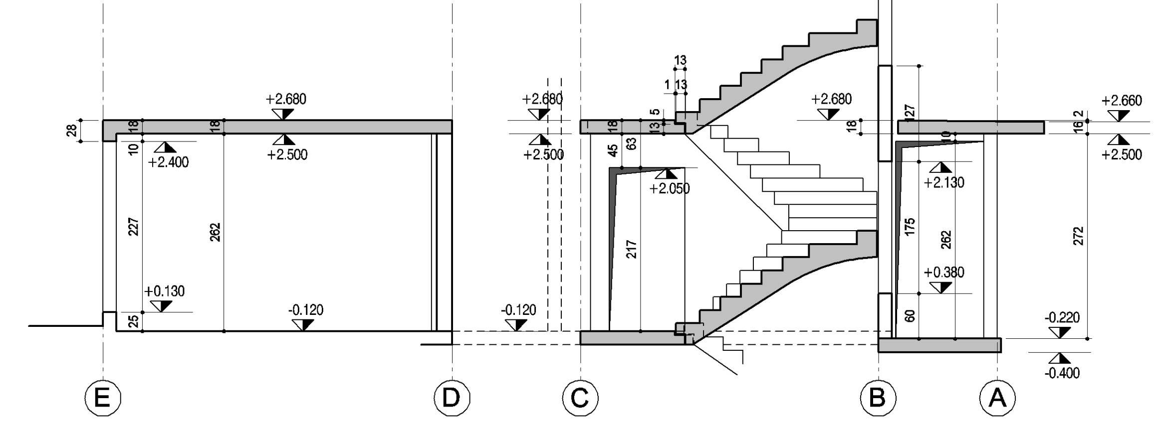
SCHNITT 2-2
