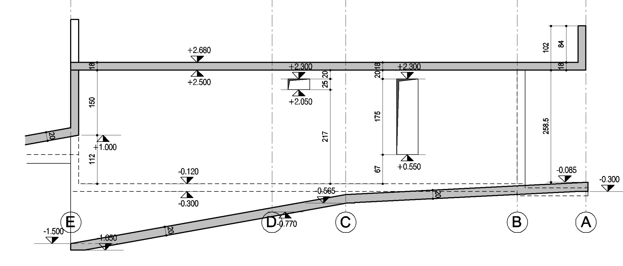
SCHNITT 3-3
