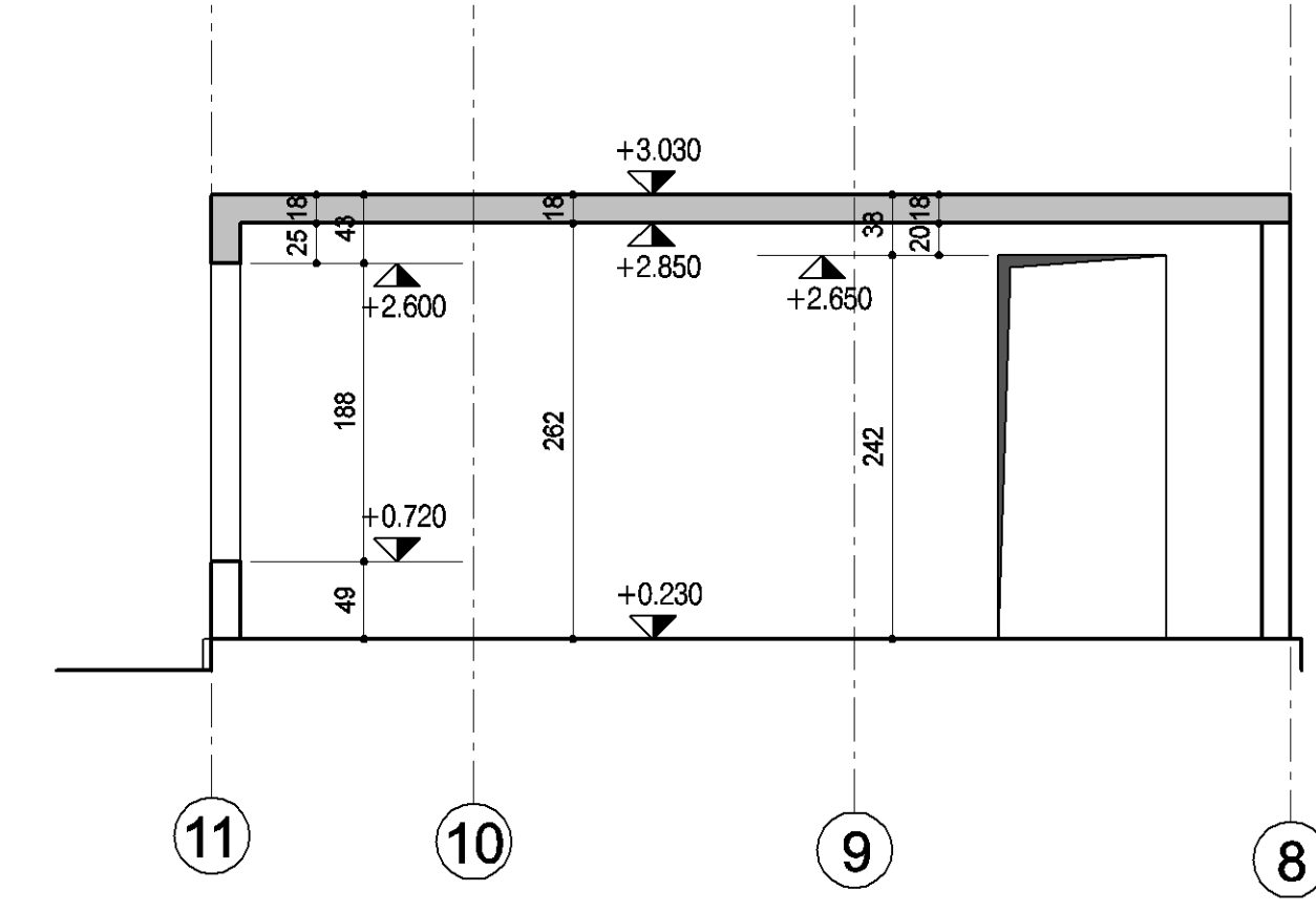
SCHNITT 5-5
